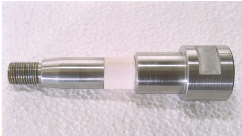
Рисунок 1 – Общий вид восстановленного наконечника центробежного молочного насоса
