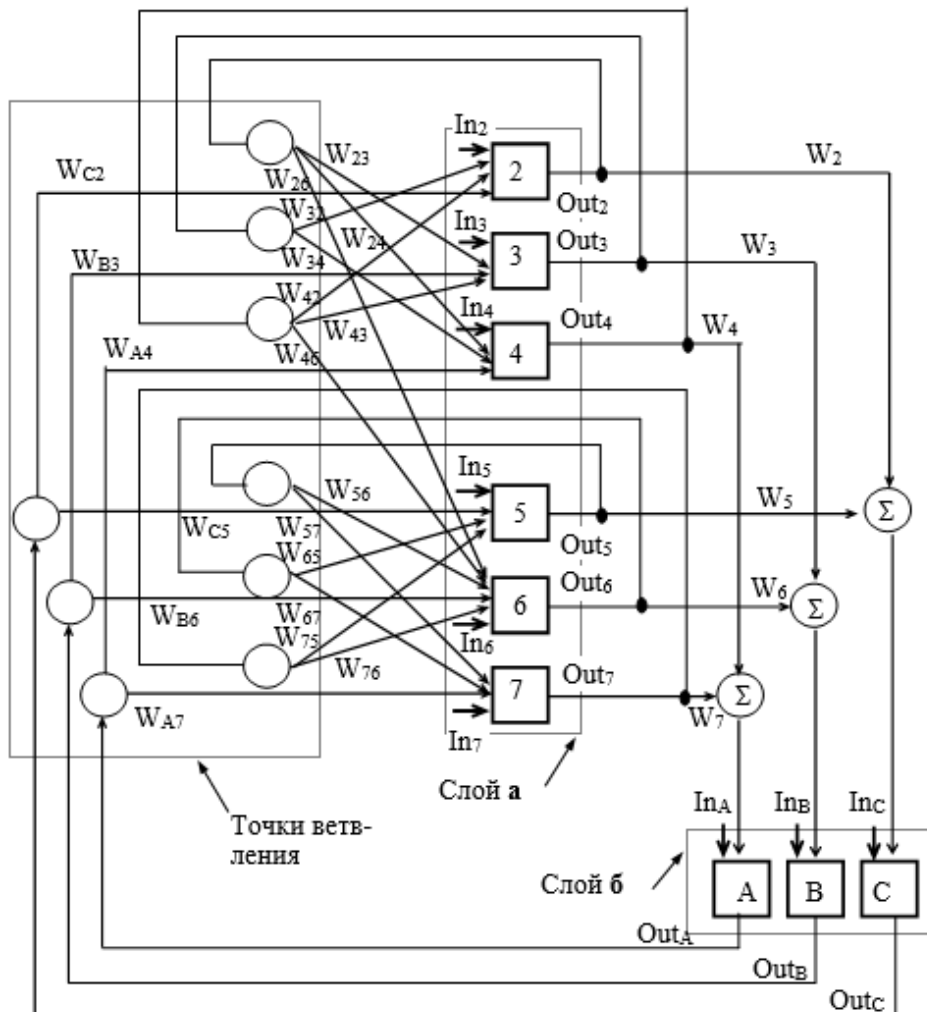
Рис. 1. Структура ИНС для оптимизации ПТП
