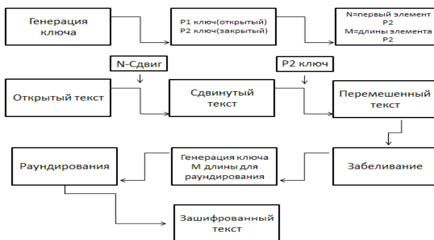
Рисунок.1 Схема гибридного шифрования
