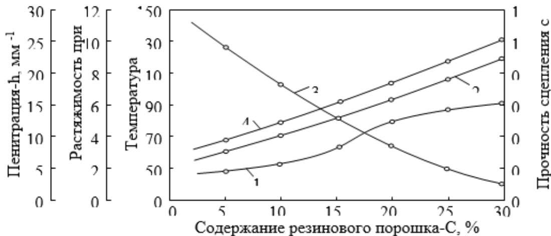
Рис. 2. Зависимость температуры размягчения (1), растяжимости при 25°C (2), пенитрации (3) и прочности сцепления с бетоном (4) композиционной мастики от содержания резинового порошка.
