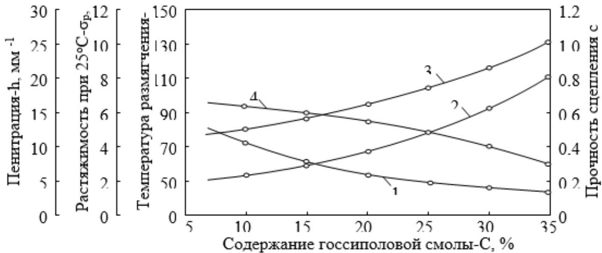
Рис. 1. Зависимость температуры размягчения (1), растяжимости при 25°C (2), пенитрации (3) и прочности сцепления с бетоном (4) композиционной мастики от содержания госсиполовой смолы.
