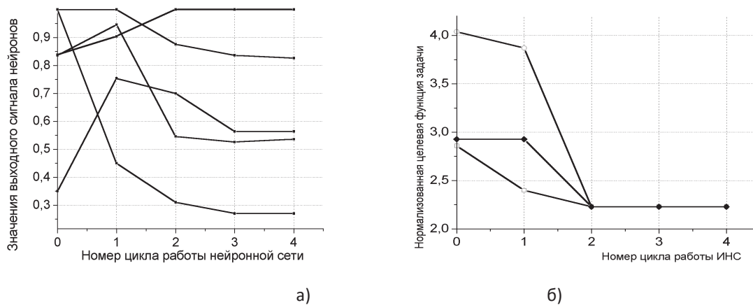
Рис.2 Графики функций, иллюстрирующие ход работы ИНС
