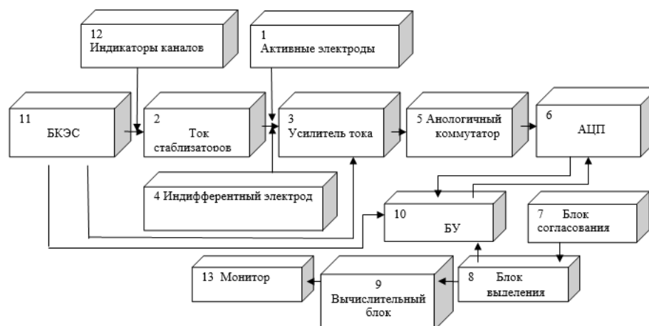
Рисунок 5. Функциональная блок-схема ММАНГ.
